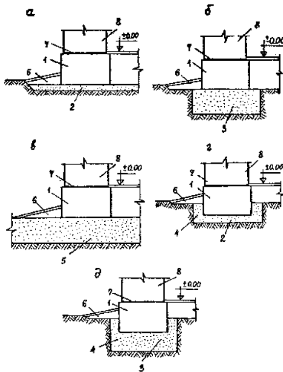
Рис.2. Конструктивные решения фундаментов;
